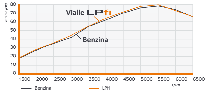
Grafico potenza LPfi / benzina
